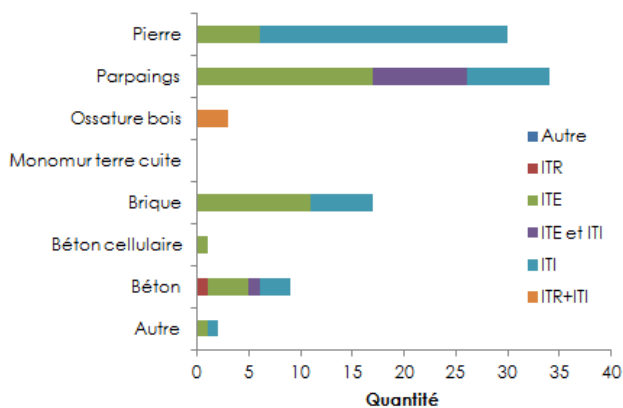
Figure 19 : Solutions de rénovation sur les murs extérieurs des maisons individuelles
