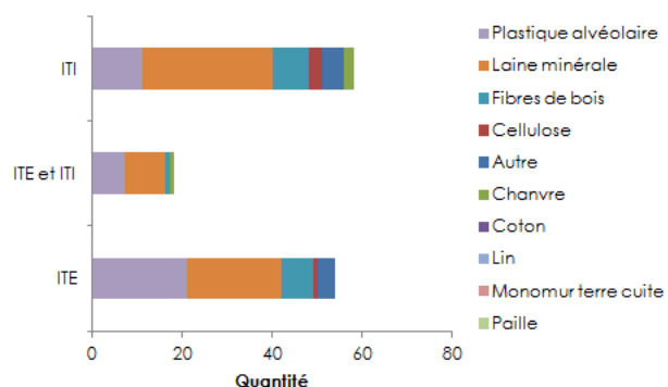
Figure 35 : Figure 36 : Isolants mis en œuvre suivant les types d'isolation en tertiaire
