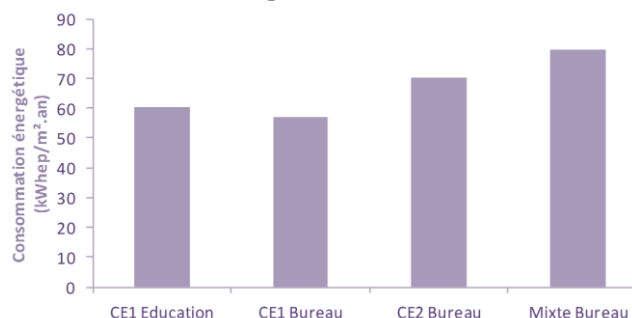
Figure 16 : Consommation réglementaires en tertiaire suivant l'usage et la présence d'un système de refroidissement
