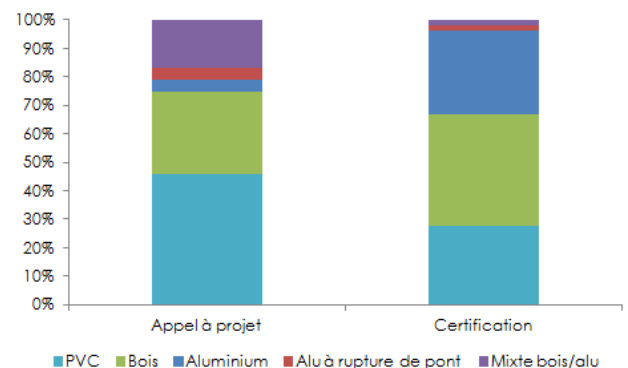
Figure 25 : Répartition des baies suivant l'origine du projet en logements individuels
