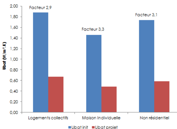
Figure 5 : Déperditions énergétiques (Ubat) avant/après travaux
