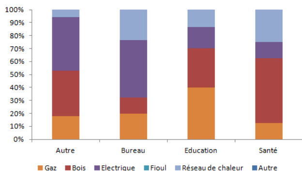
Figure 55 : Répartition de l'énergie de chauffage après travaux dans les bâtiments tertiaires suivant leurs usages
