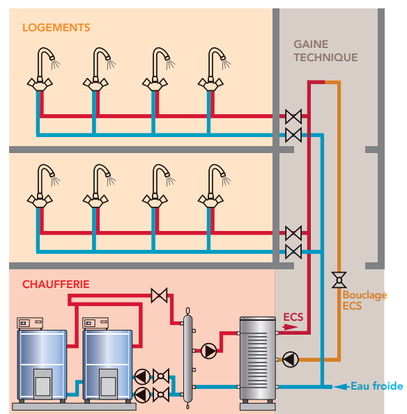
Figure 3 : Découpage d'une installation d'ECS suivant les trois niveaux définis dans la RT 2012
