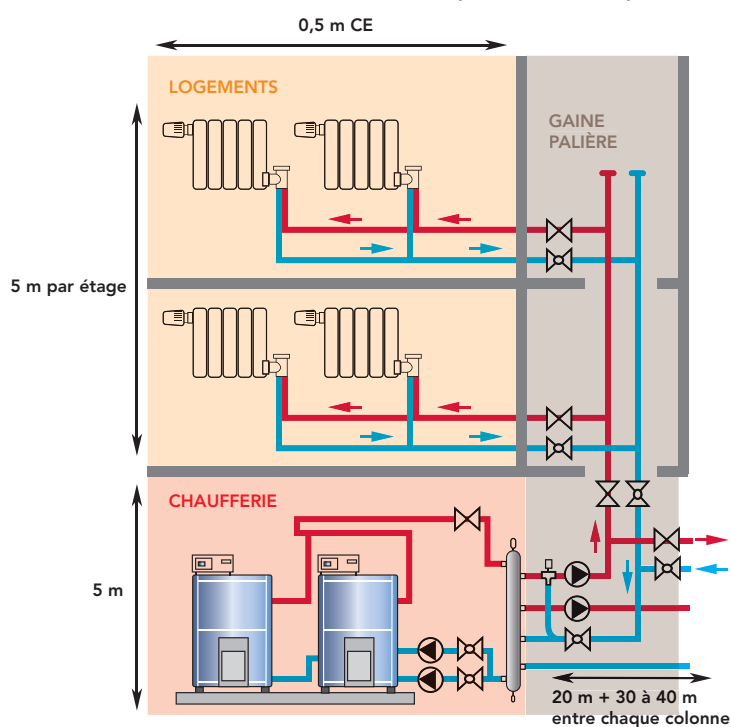
Figure 8 : Les longueurs à prendre en compte
