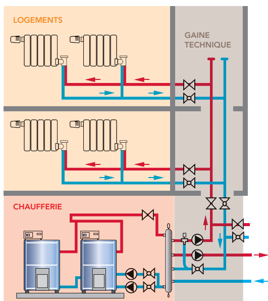
Figure 2 : Découpage d'une installation de chauffage suivant les trois niveaux définis dans la RT 2012
