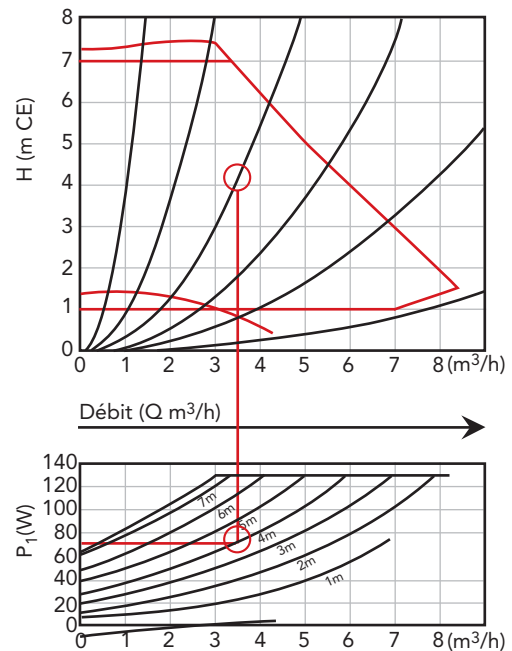
Figure 9 : Exemple de détermination de la puissance électrique d'un circulateur
