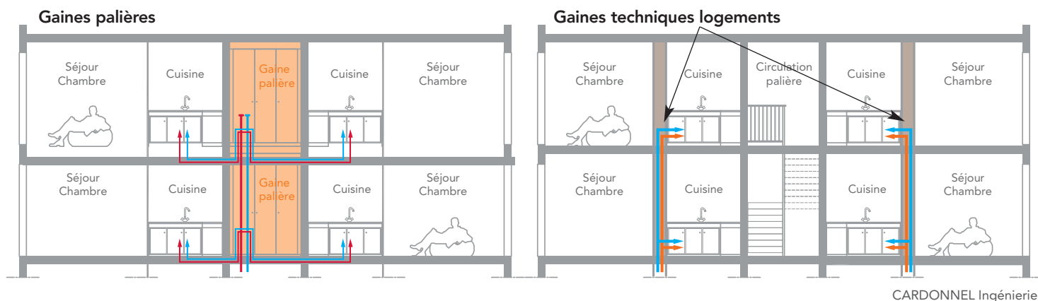
Figure 6 : Les distributions en gaine palière (à gauche) et en gaine technique logement (à droite) sont deux configurations présentes dans les immeubles d'habitations collectives
