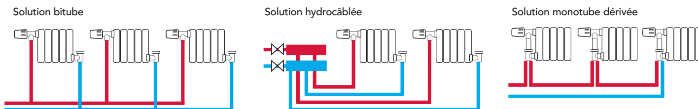
Figure 4 : Les trois principes d'alimentation des radiateurs
