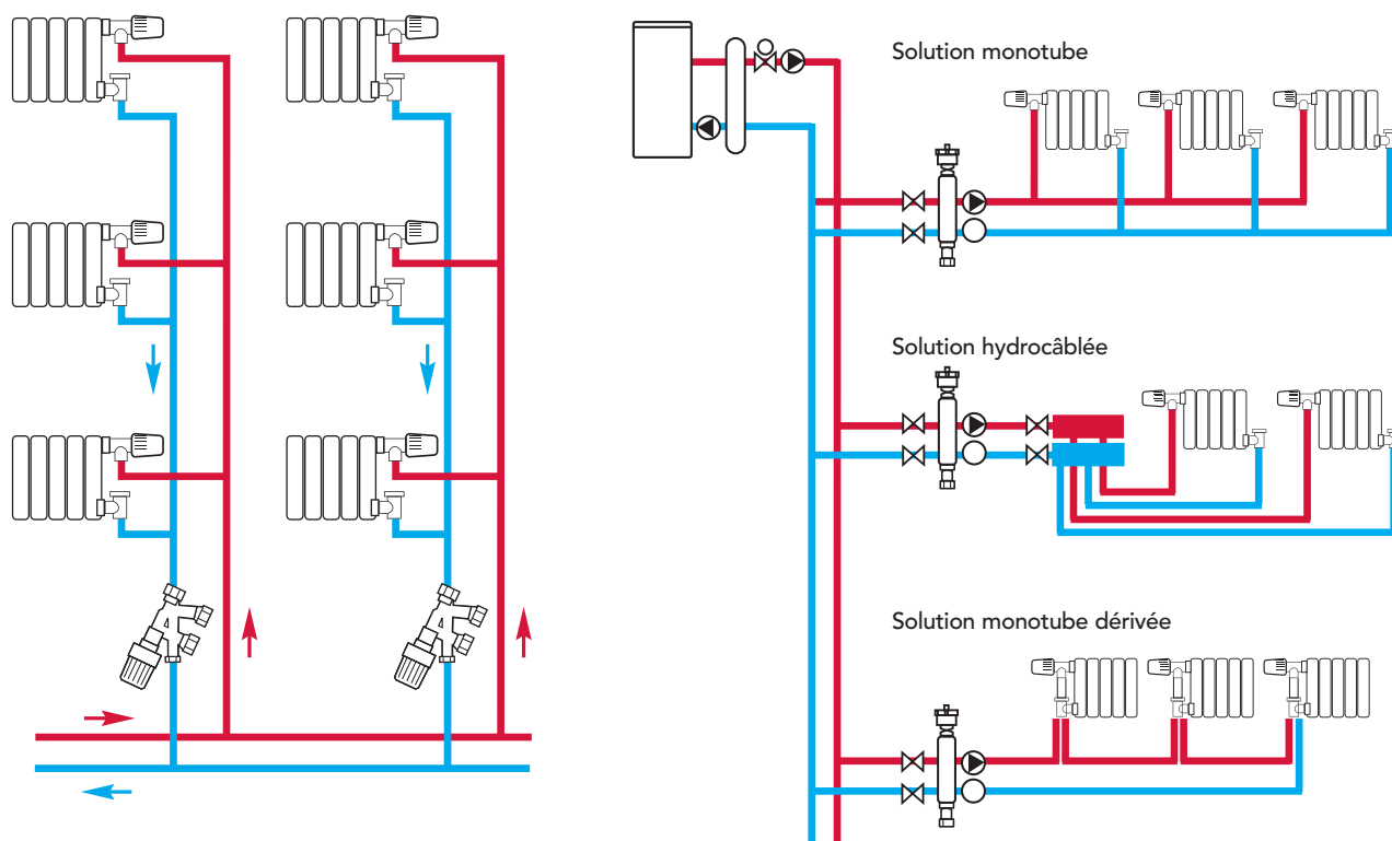
Figure 5 : Schémas de principe d'une distribution par colonnes montantes (à gauche) et Chauffage Individuel Centralisé (CIC, à droite)
